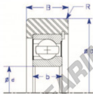
Max-Type
